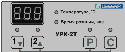
Рис.1 Вид передней панели УПК-2Т.
