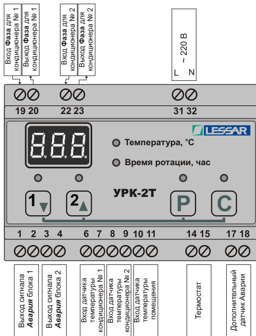
Рис.2 Схема подключения.
